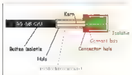
Typische opbouw krimconnector.
